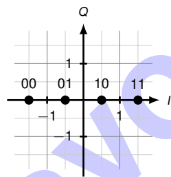
Abbildung 5.1: Signalraumkonstellation
