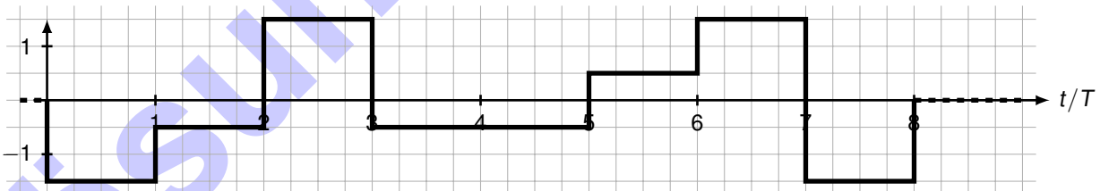
Abbildung 5.2: Basisbandsignal
